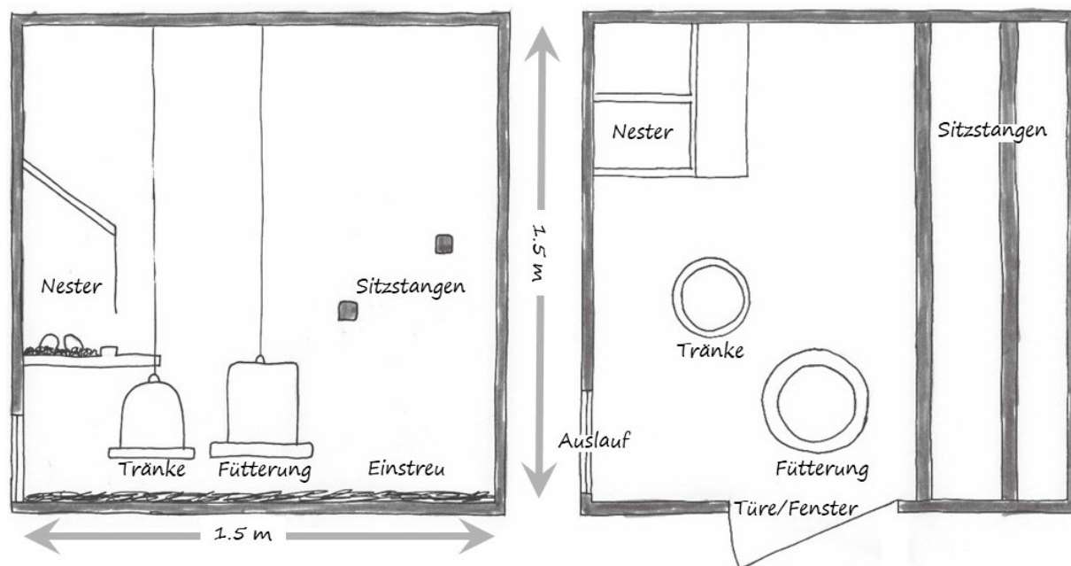
Abbildung 1: Beispiel eines Stalls mit den erforderlichen Einrichtungen für die Haltung von Gruppen bis zu 8 Hühnern. Die Sitzstangen müssen auf verschiedenen Höhen angebracht sein, mindestens 50 cm über dem Boden und mit mindestens 50 cm Freiraum darüber. Für jeweils fünf Hühner muss mindestens ein Nest angeboten werden. Der Boden muss mit Einstreu bedeckt sein.
